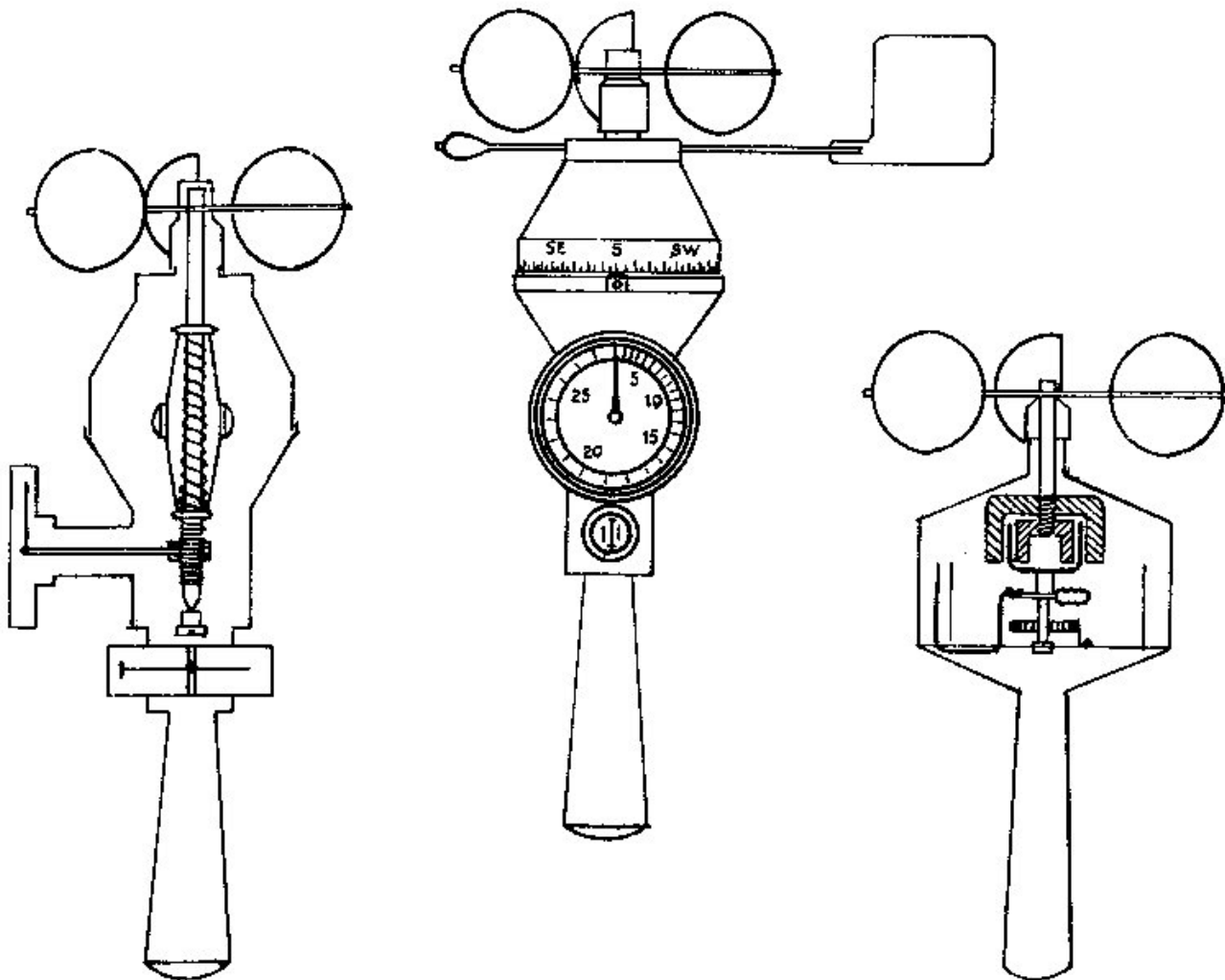
Fig. 4.15 - Anemometri a mano.
