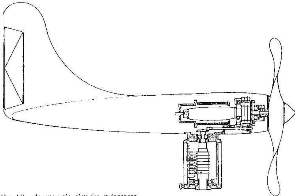
Fig. 4.7 - Anemografo elettrico autogeneratore: trasmettitore.
