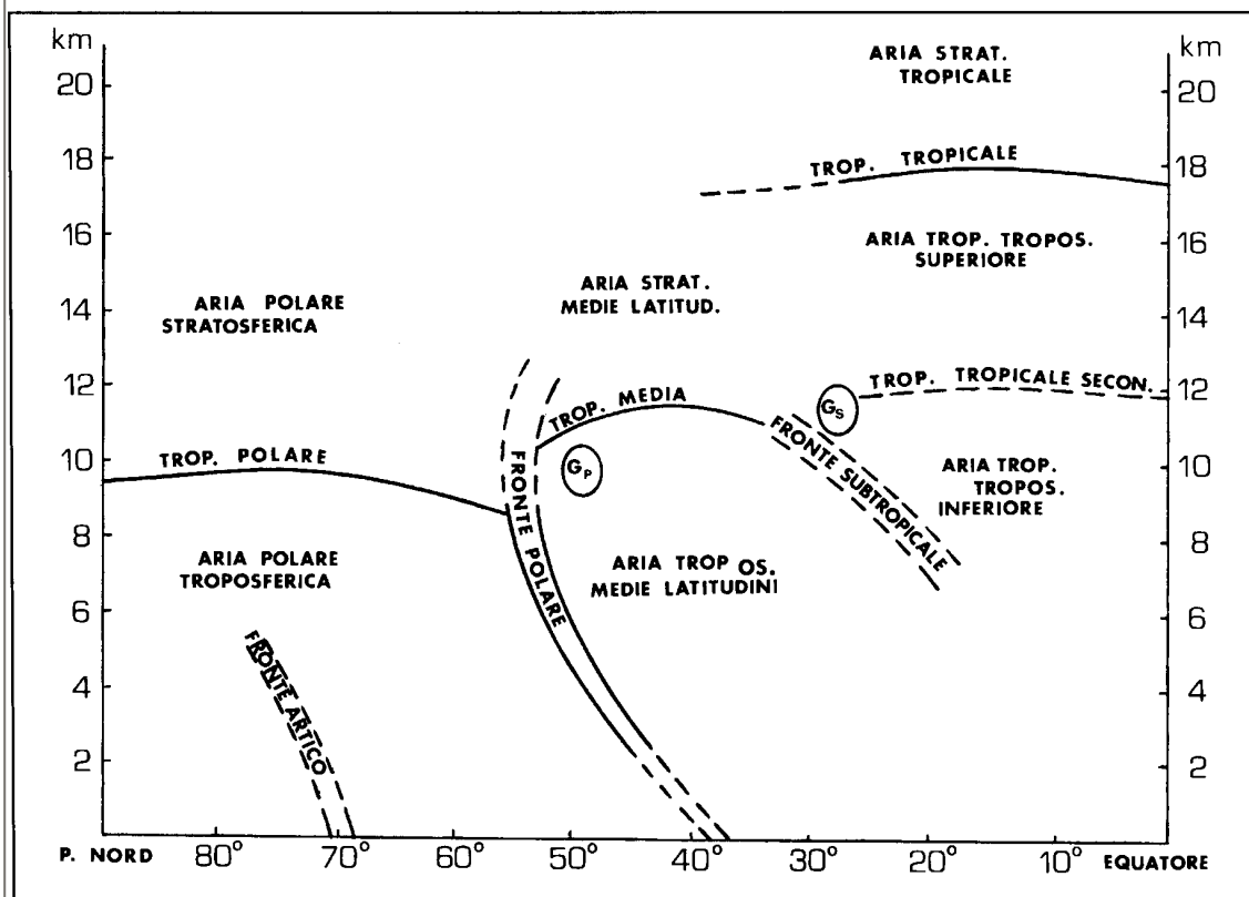
Fig. 5 Principali masse d'aria, tropopausa, fronti e correnti a getto, in relazione ai sistemi di vento nei bassi strati. I fronti possono essere ben sviluppati o relativamente deboli, in relazione ai diversi periodi dell'anno e alle regioni geografiche.
