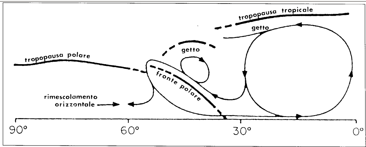
Fig.6 Modello di circolazione a tre celle dovuto a Palmen (1951)
