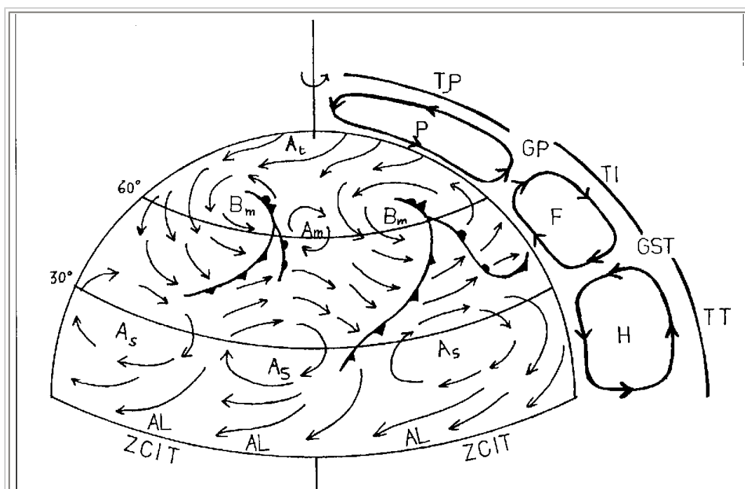
Fig. 3 Circolazione generale dell'atmosfera a tre celle: di Hadley (H), di Ferrel (F) e Polare (P). Sono segnalate le posizioni del getto subtropicale (GST) e di quello polare (GP), della tropopausa tropicale (TT), intermedia (TI) e polare (TP), degli anticiclони subtropicali ( A_s ) e di quelli termici polari ( A_t ), delle alte e basse mobili delle medie latitudini ( A_m e B_m ), degli alisei (AL) e della zona di convergenza intertropicale (ZCIT)
