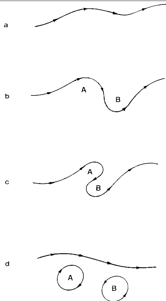
Fig. 5 Fasi del ciclo ondulatorio delle configurazioni di flusso in quota alle medie latitudini.
