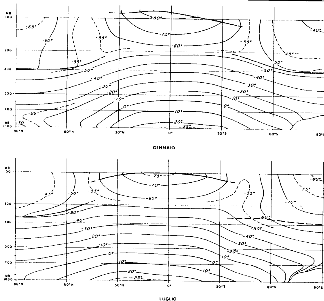
Fig. 4 Temperature in °C mediate lungo cerchi di latitudine per gennaio e luglio. Le linee più scure mostrano la posizione media delle tropopause.
